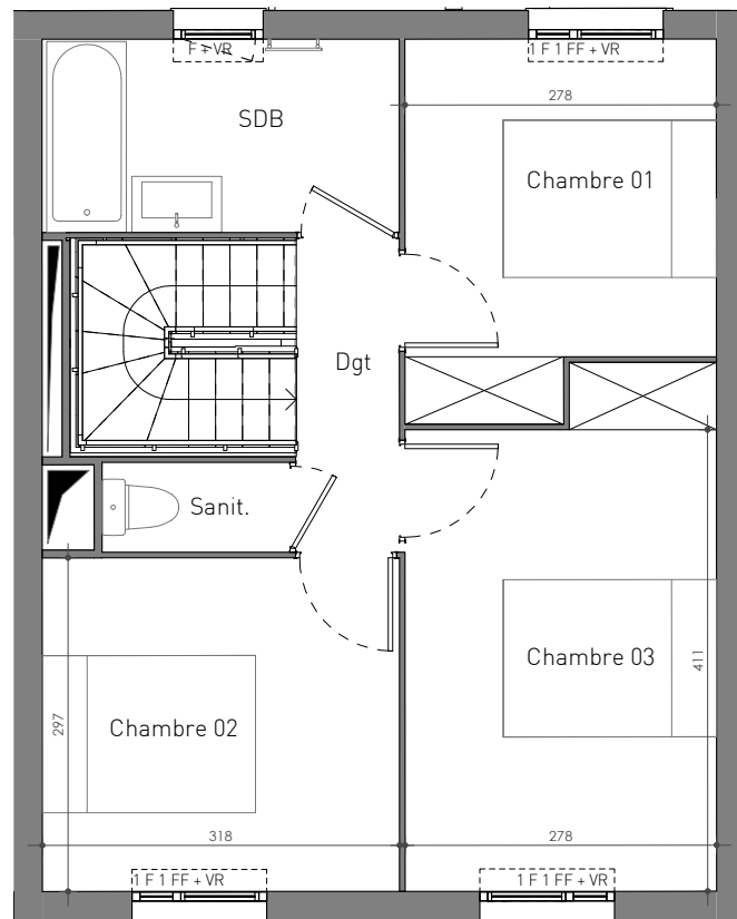
Étage
